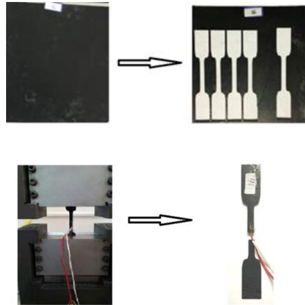
Fig. 3 Tensile Test
